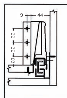
Fissaggio pannello posteriore Back panel fixing
