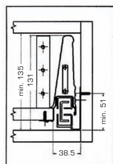
Fissaggio guide Guides fixing
