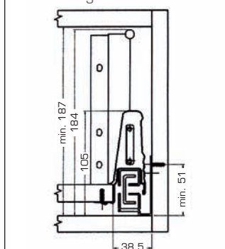
Fissaggio guide Guides fixing
