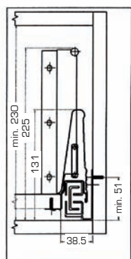
Fissaggio guide Guides fixing
