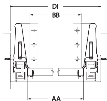
Fissaggio guide Guides fixing
