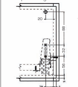
Fissaggio pannello anteriore Frontal panel fixing
