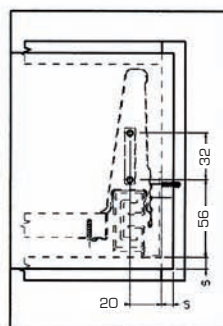
Fissaggio pannello anteriore Frontal panel fixing
