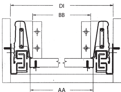
Fissaggio guide Guides fixing
