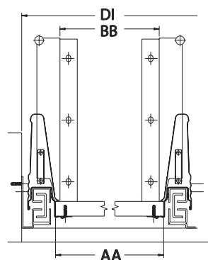
Fissaggio pannello anteriore Frontal panel fixing
