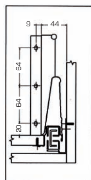
Fissaggio pannello posteriore Back panel fixing
