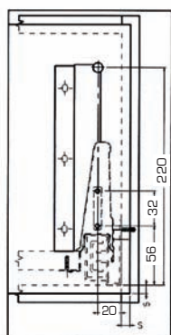
Fissaggio pannello anteriore Frontal panel fixing
