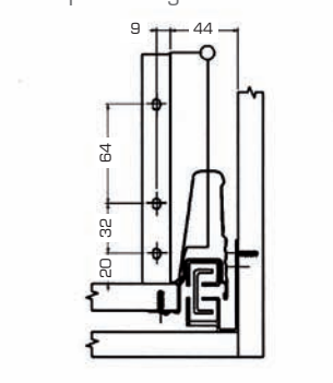
Fissaggio pannello posteriore Back panel fixing
